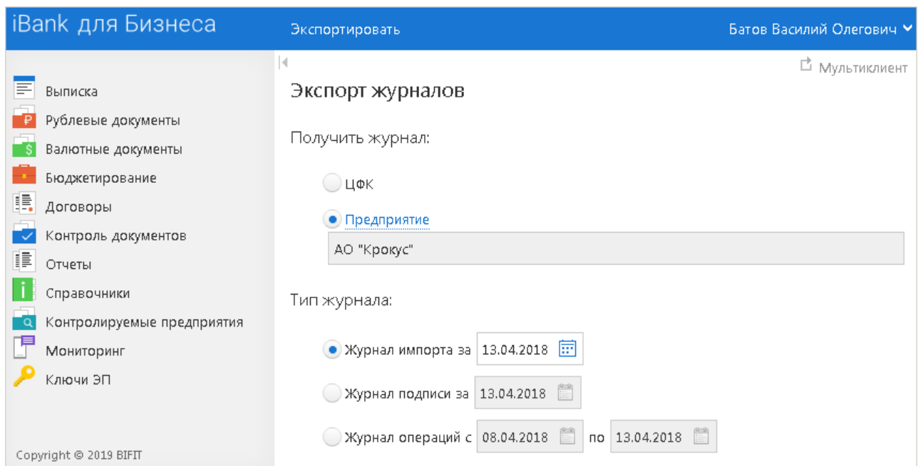
Рис. 12. Экспорт журналов
