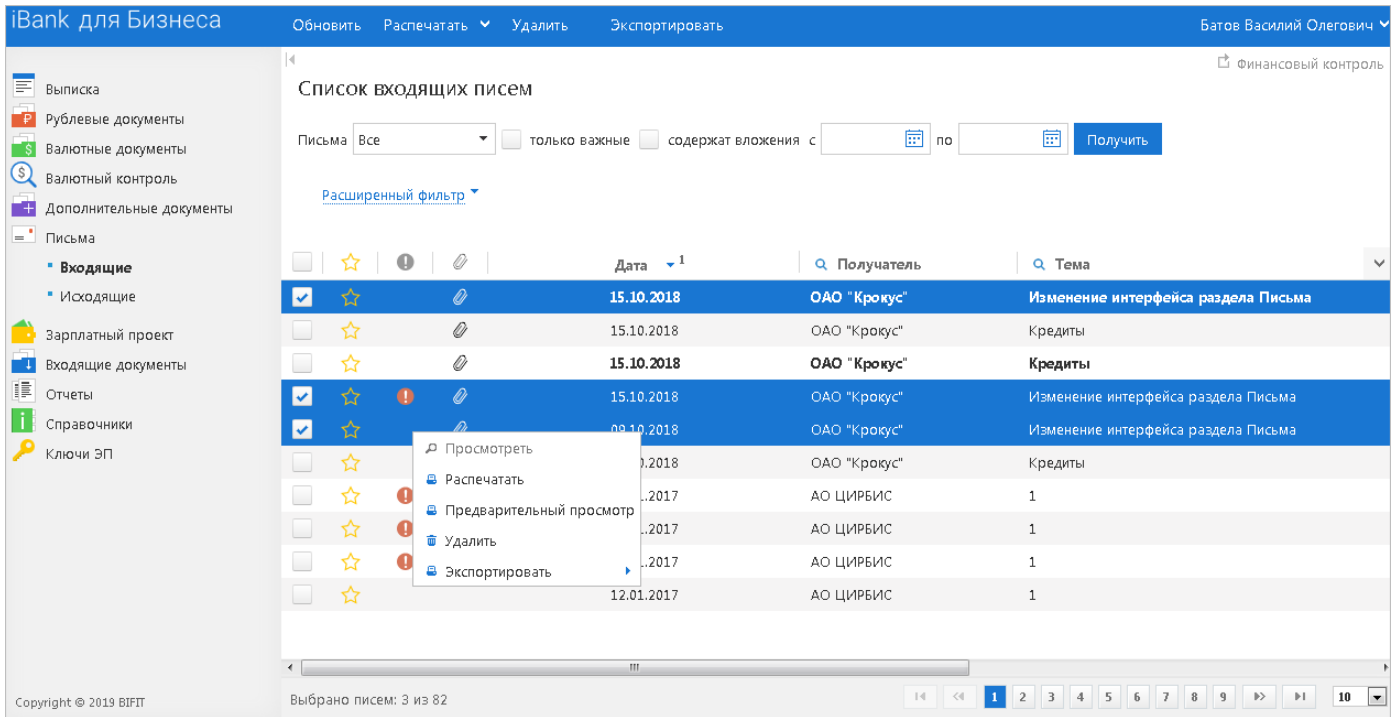
Рис. 72. Удаление писем
